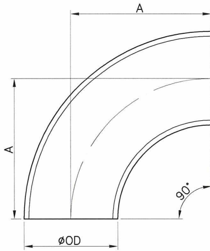
90° L-R ELBOW
