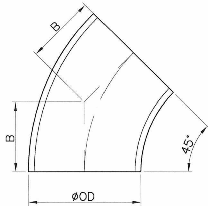
45° L-R ELBOW
